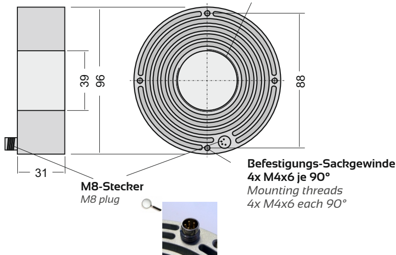
Seitenansicht im Schnitt Side view (sectional view)
